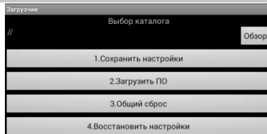
Рис. 3. Успешное подключение
